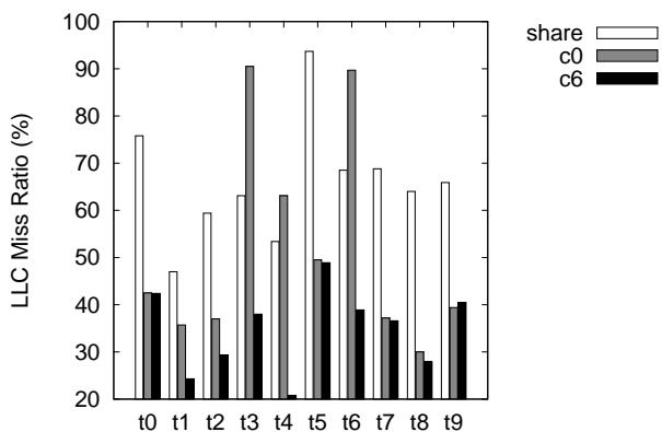
Fig. 9. CAS Evaluation
