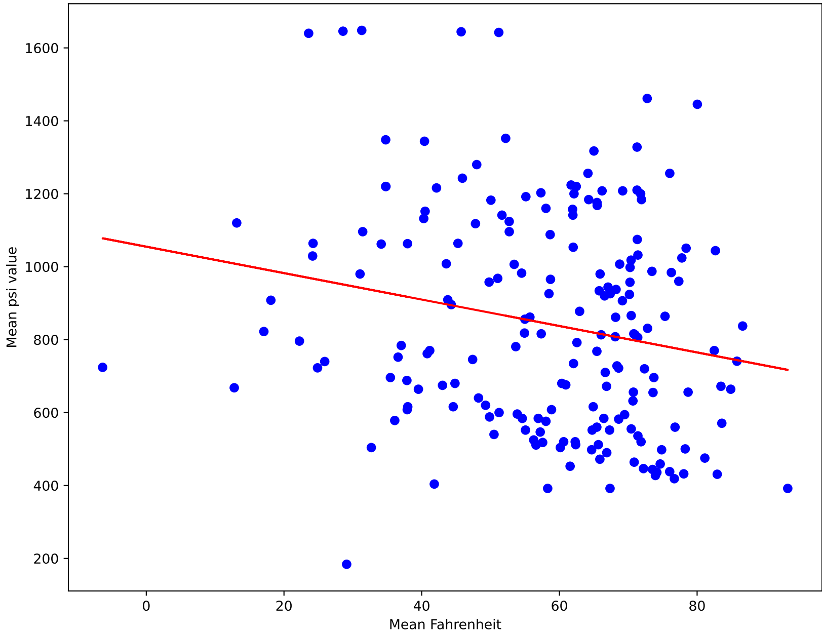
Device BU Med 815 Albany 15 Yd ( R^2=0.04 )
