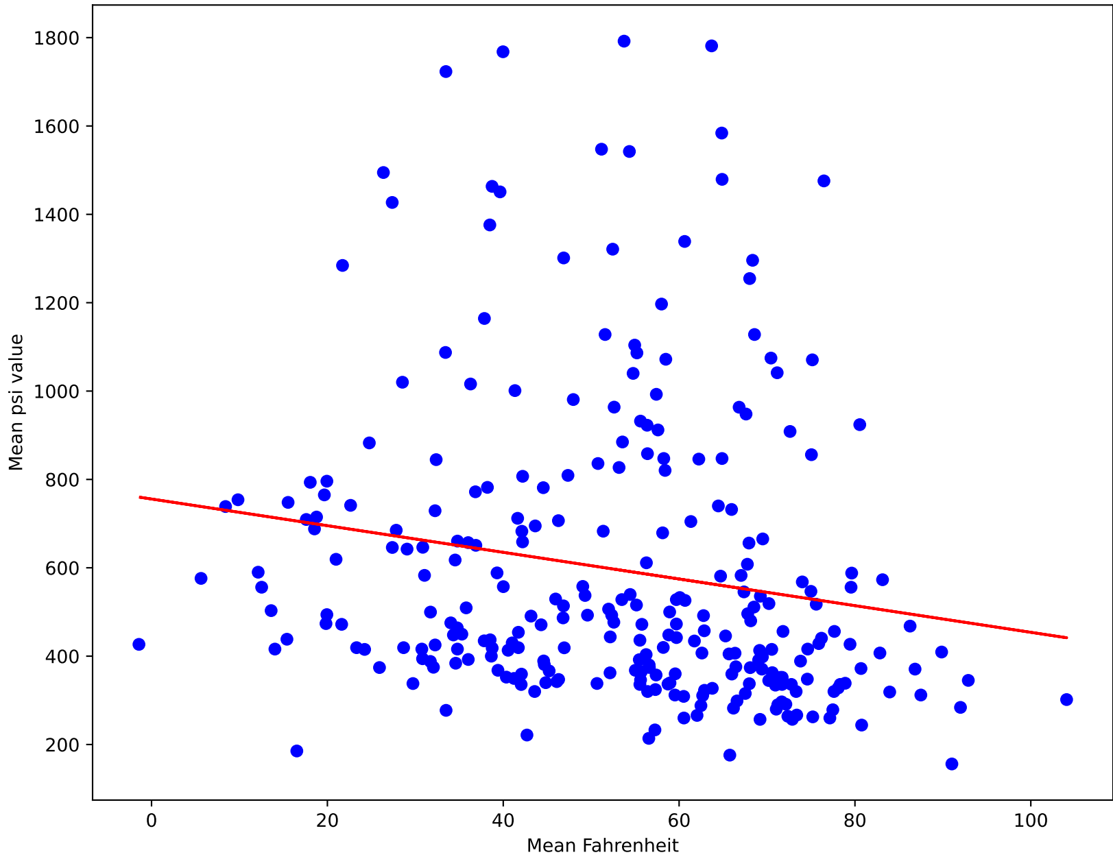
Device BU Med 700 Albany 20 Yd ( R^2=0.03 )
