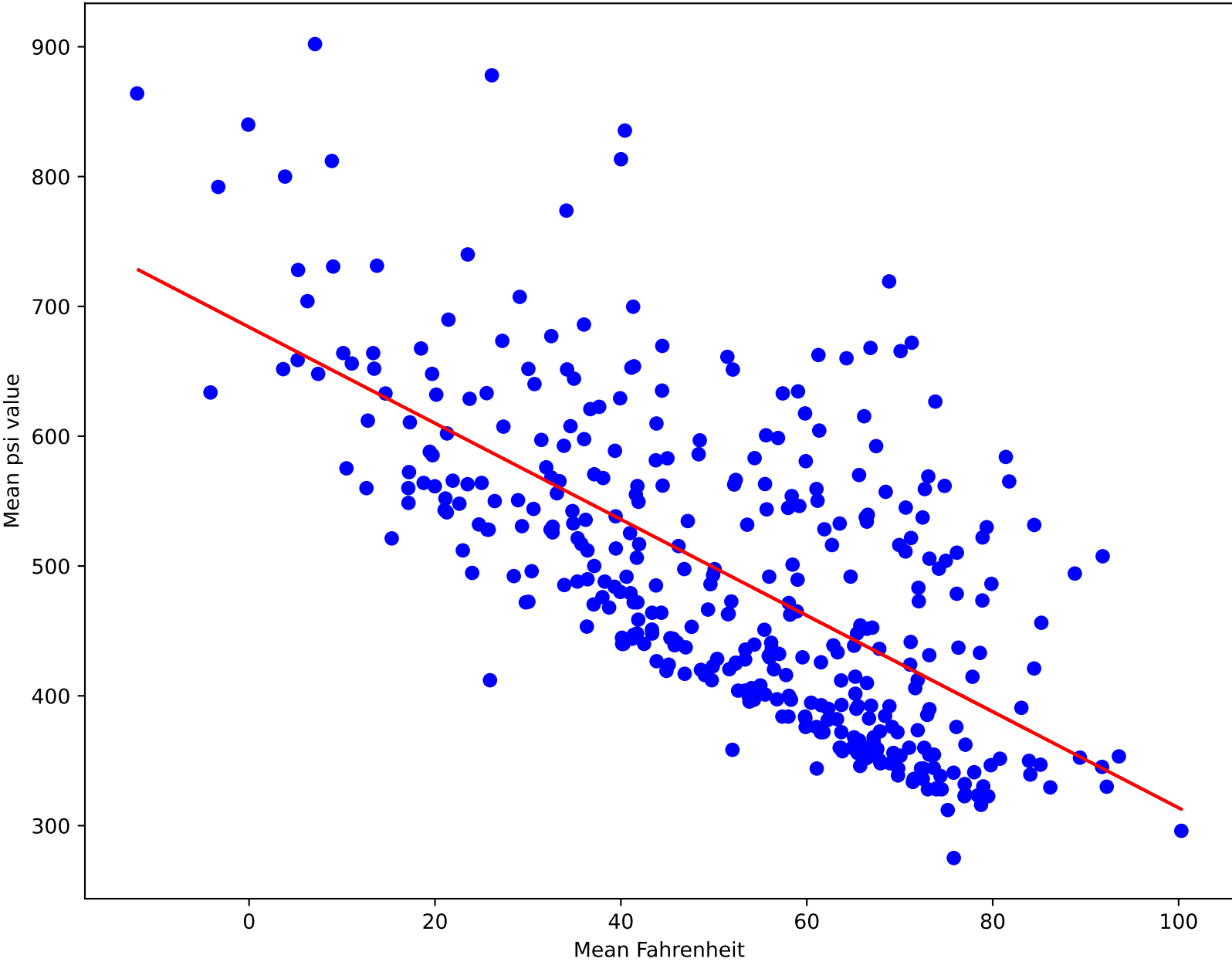
Device BU MED - 15 Stoughton 35 Yd ( R^2=0.44 )
